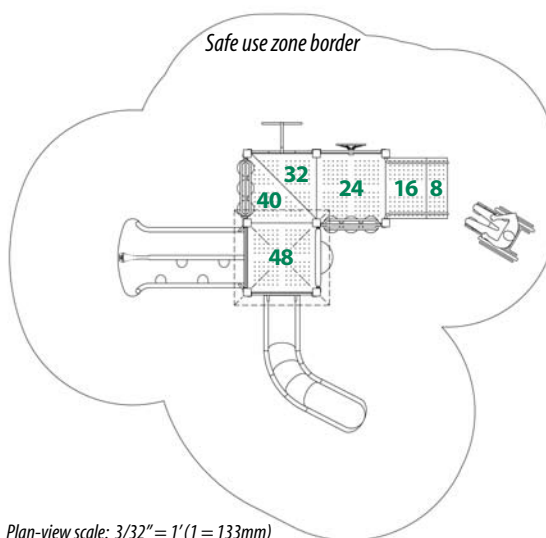
Plan-view scale: 3/32" = 1' (1 = 133mm)
